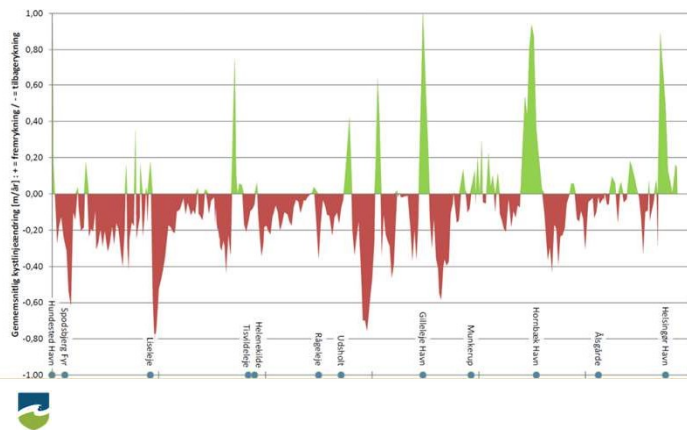
Kystlinjeændring mellem år 1897 og 2003 på Nordkysten
